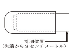
<ちくとうの最小直径値の計測方法>
