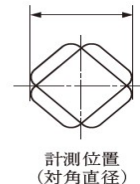
<ちくとうの最小直径値の計測方法>
