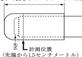
<竹刀の先革長、先端部最小直径値の計測方法>
